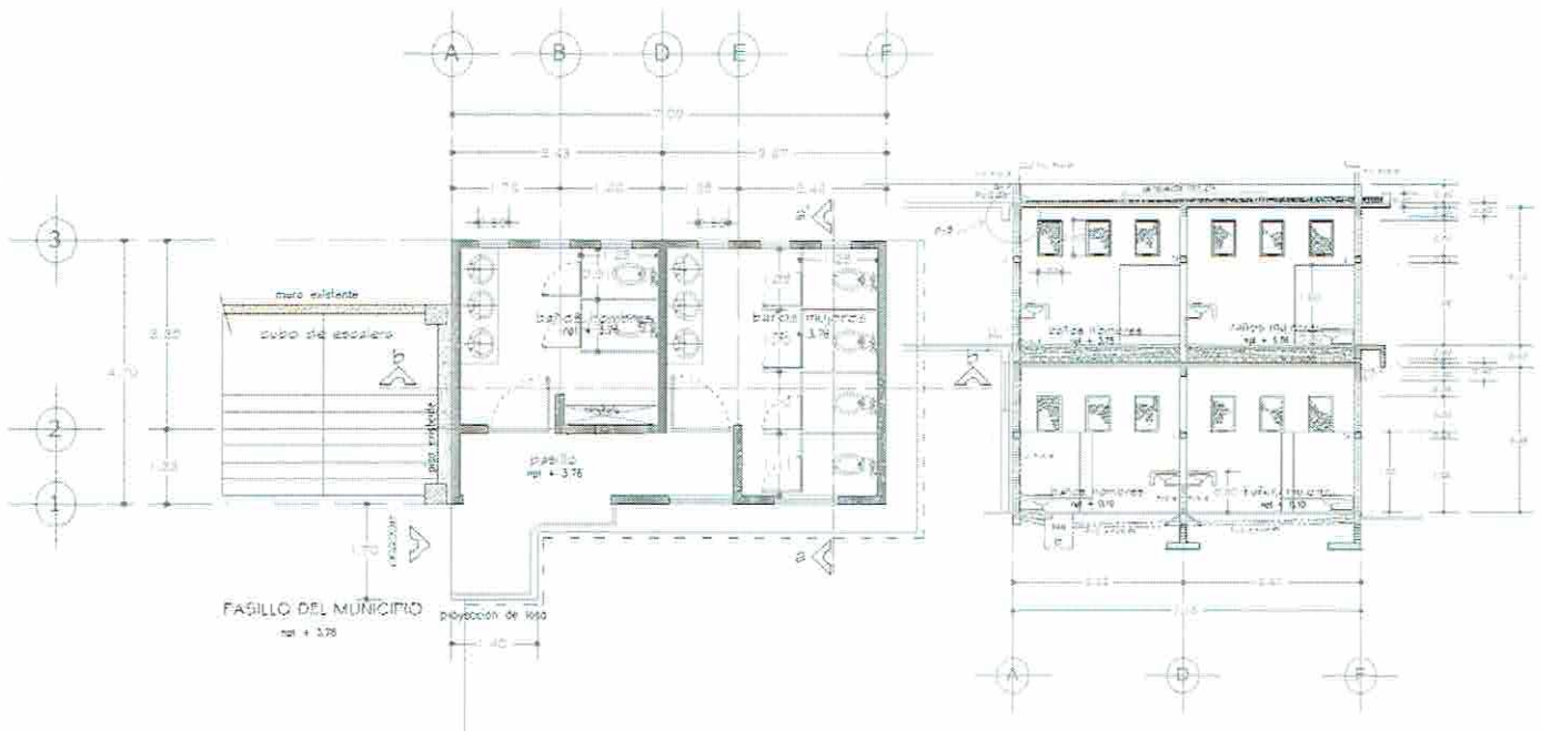
PLANTA ARQUITECTONICA ALTA
