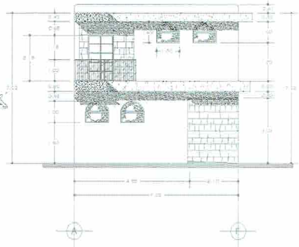
FACHADA ORIENTE
