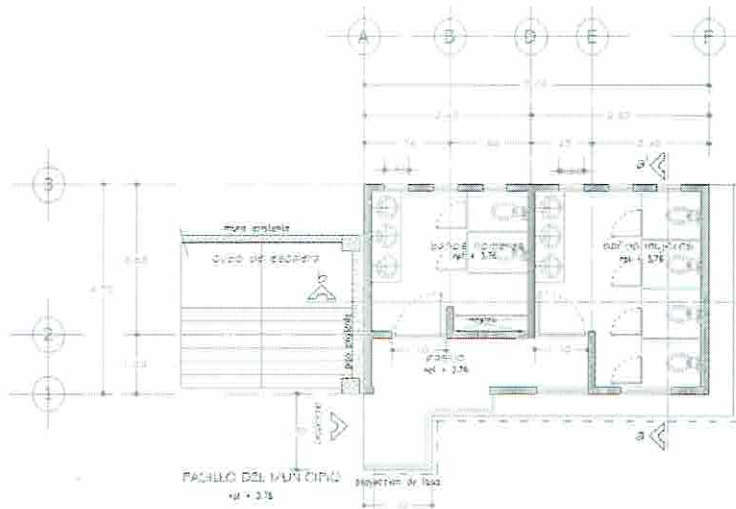
PLANTA ARQUITECTONICA ALTA
