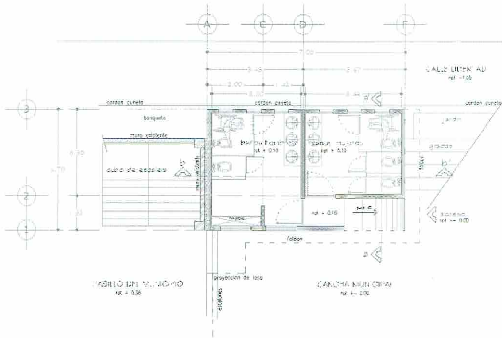
PLANTA ARQUITECTONICA BAJA
