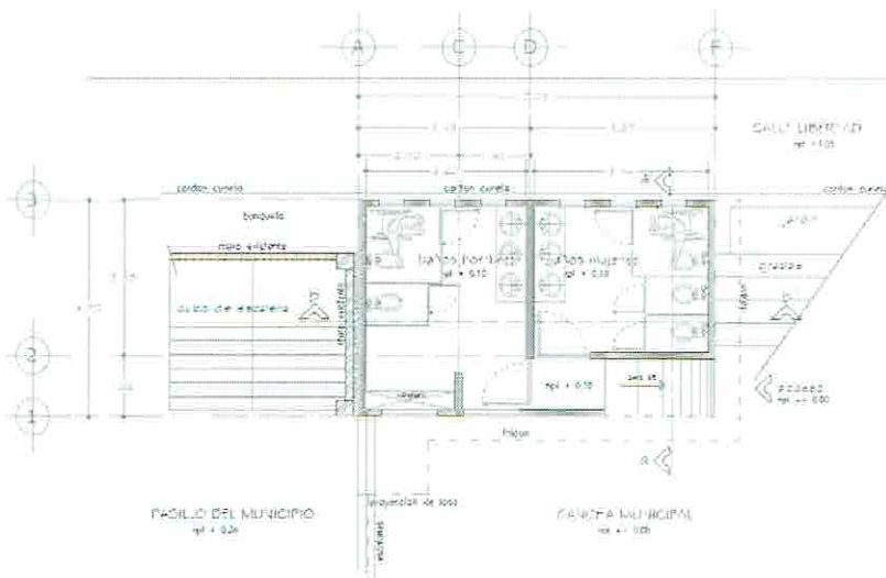
PLANTA ARQUITECTONICA BAJA
