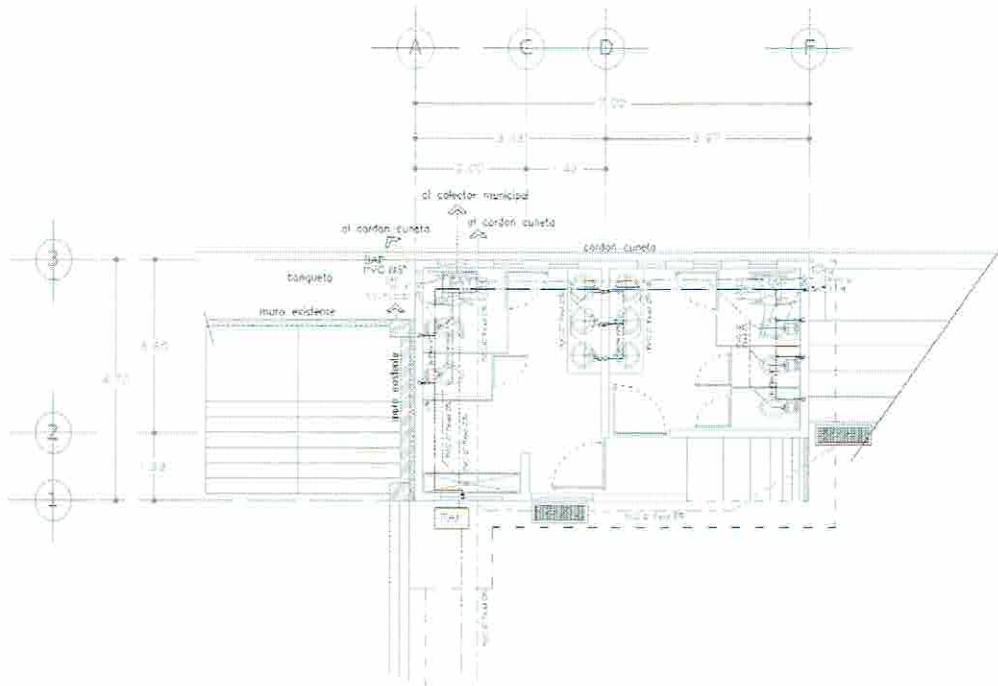
PLANTA ARQUITECTONICA BAJA Instalacion Hidrosanitaria
