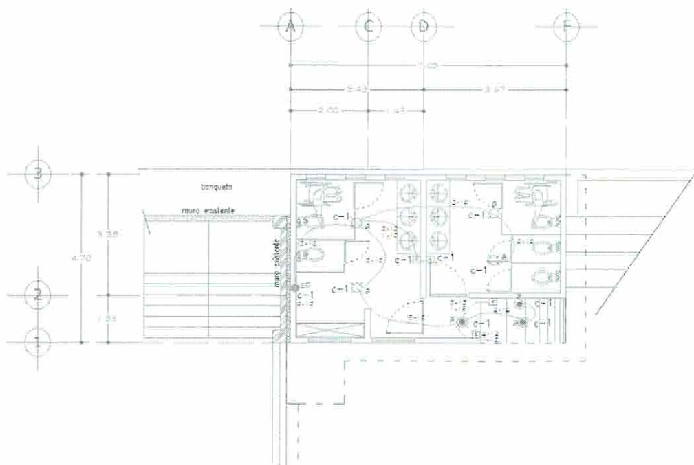
PLANTA ARQUITECTONICA BAJA Instalacion Electrica
