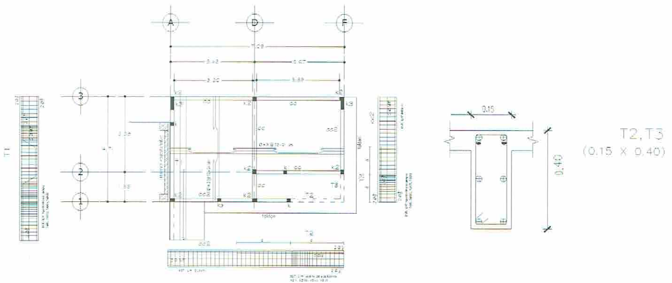
ESTRUCTURAL DE ENTREPISO
