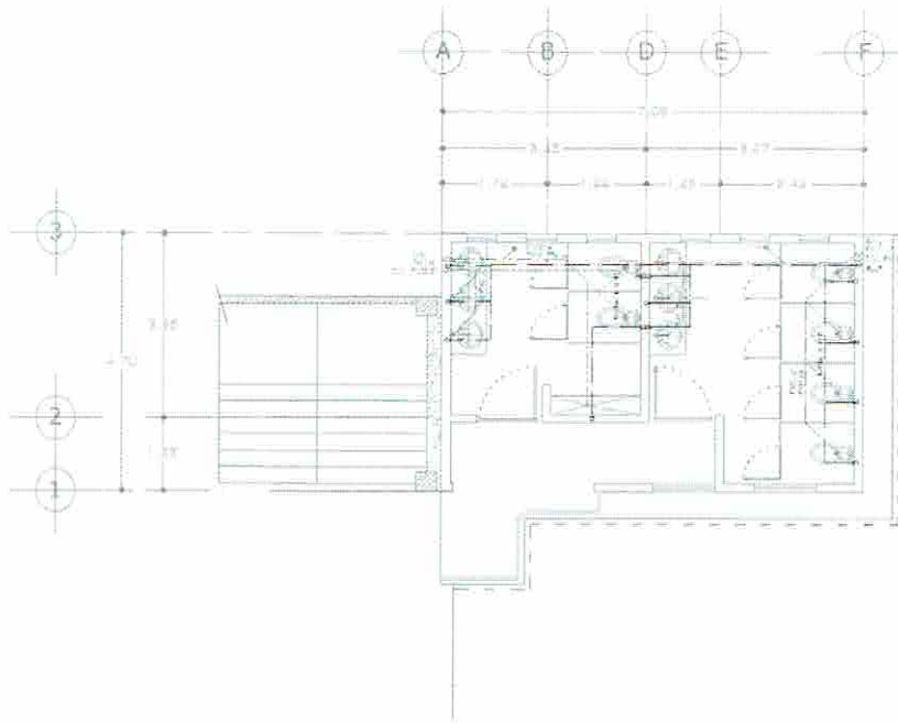
PLANTA ARQUITECTONICA ALTA Instalacion Hidrosanitaria
