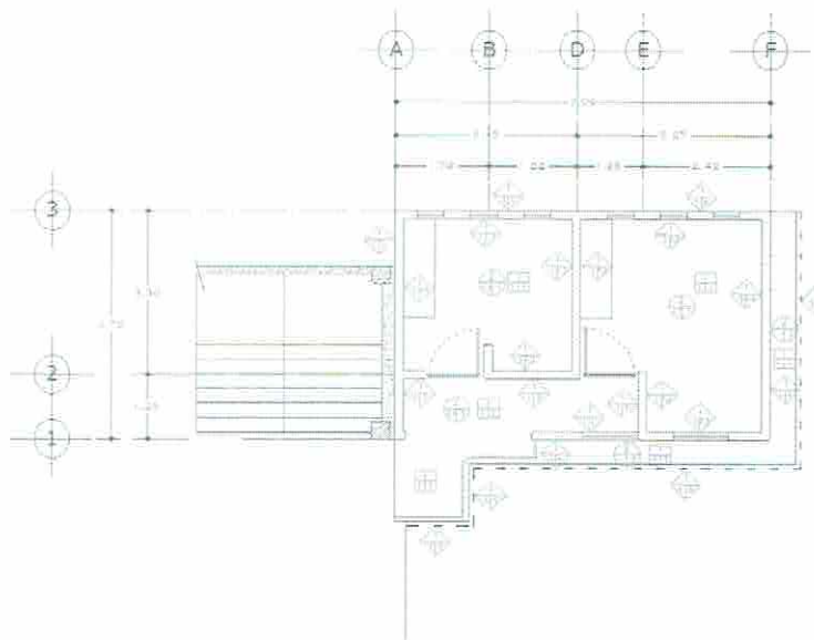
PLANTA ARQUITECTONICA ALTA Acabados
