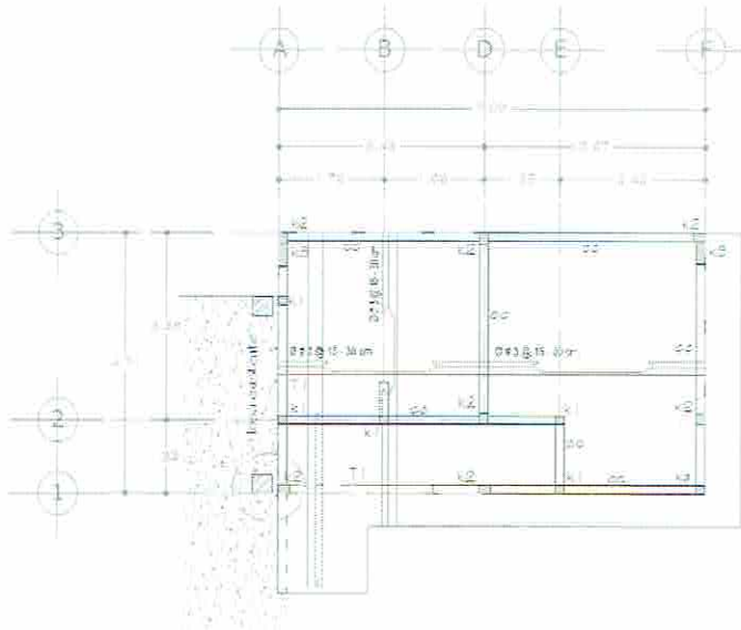
ESTRUCTURAL DE AZOTEA
