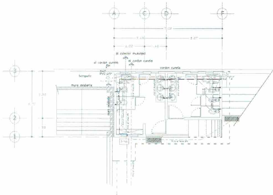
PLANTA ARQUITECTONICA BAJA Instalacion Hidrosanitaria
