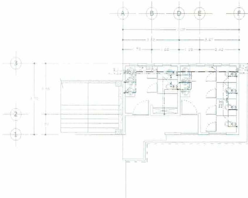
PLANTA ARQUITECTONICA ALTA Instalacion Hidrosanitaria
