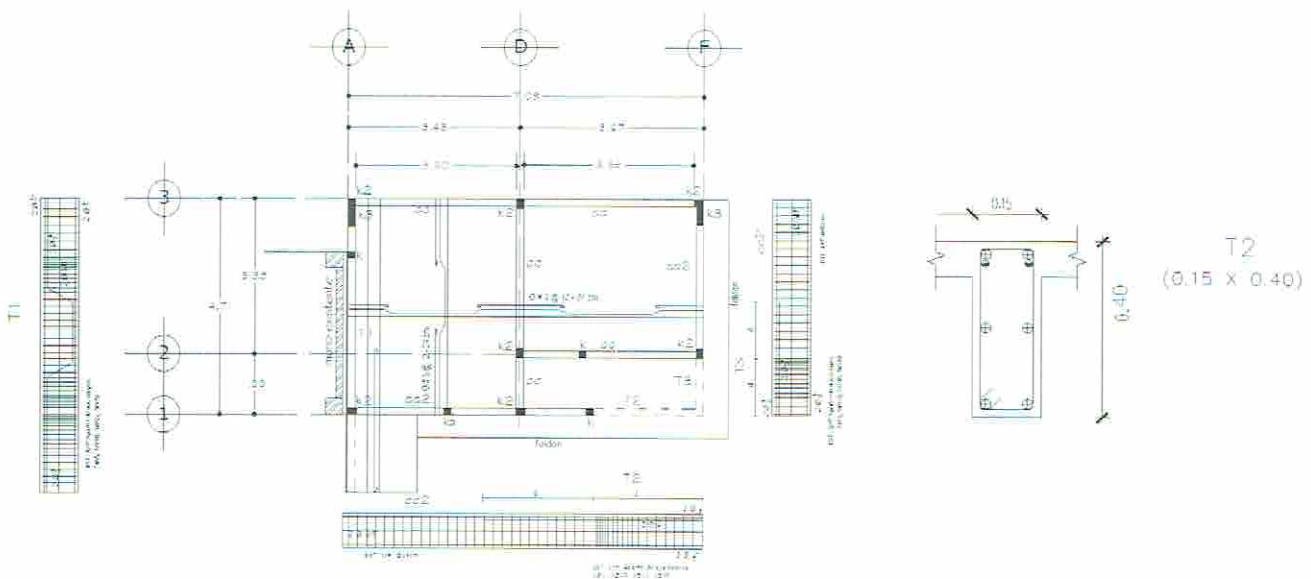
ESTRUCTURAL DE ENTREPISO
