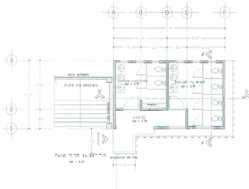
PLANTA ARQUITECTONICA ALTA
