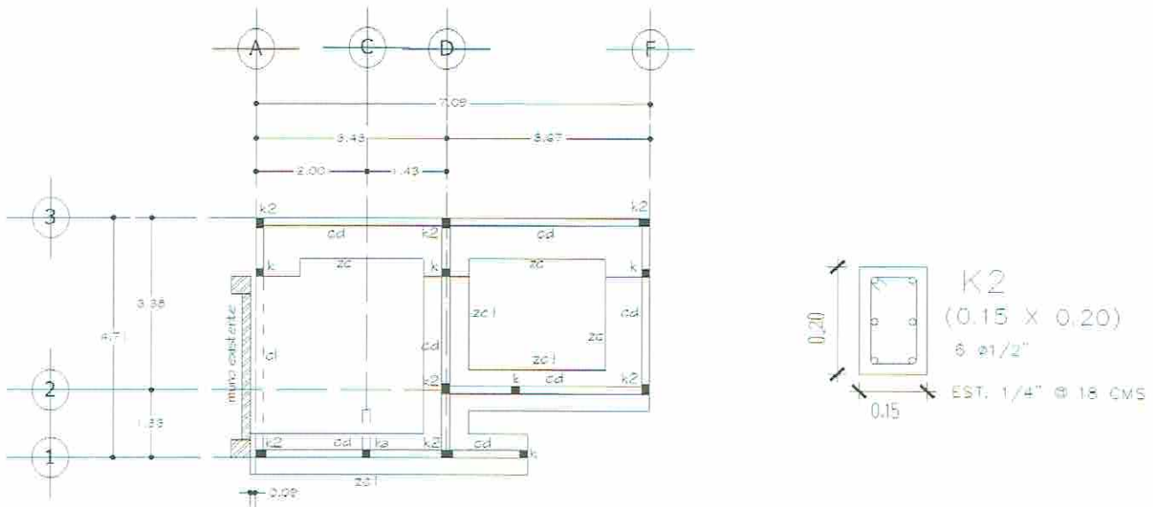
PLANTA DE CIMENTACION
