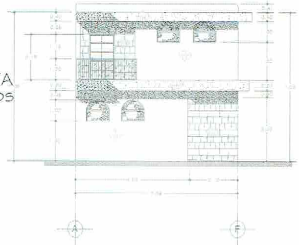
FACHADA ORIENTE Acabados
